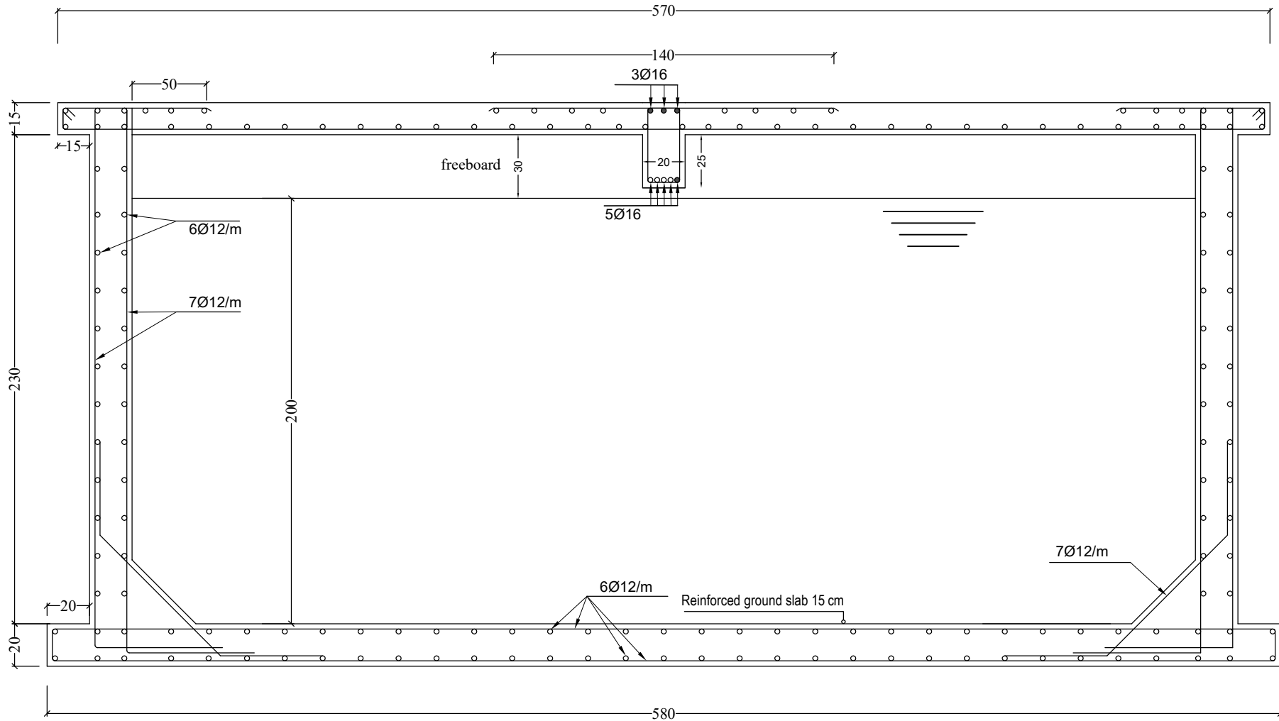
Reinforcement detail in long direction تفاصيل التسليح بالاتجاه الطويل 1/25
