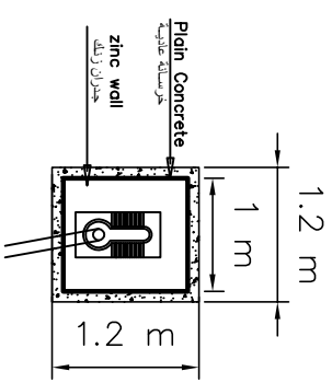
مقطع أفقي Top view
