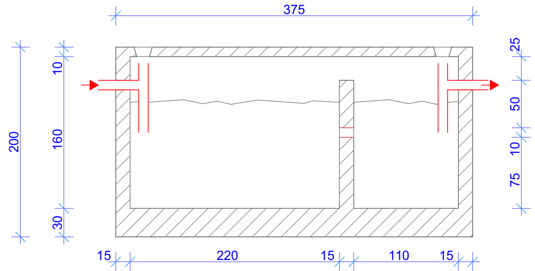
COUPE
