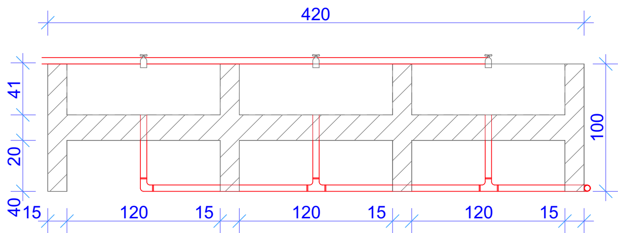
COUPE LONGITUDINALE
